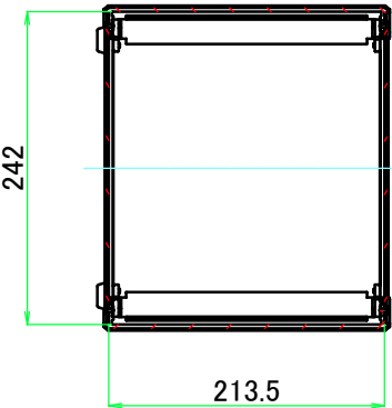
A-A ( 1 : 6.5 )
